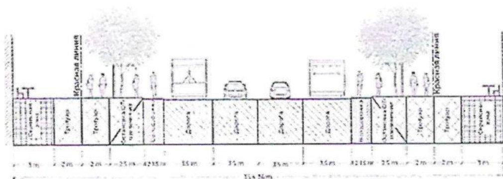
Магистральная улица районного значения тип 3
