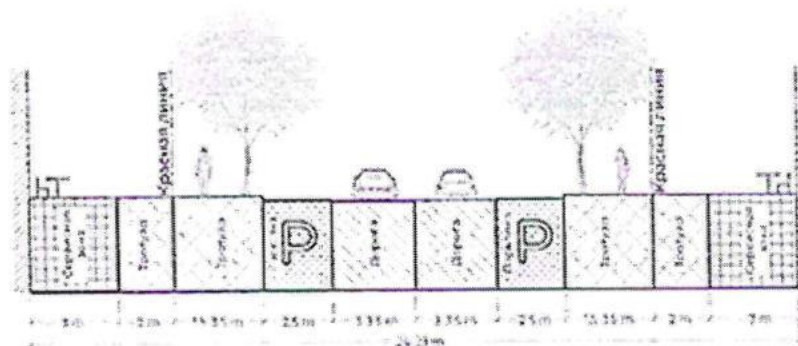
Улицы и дороги местного назначения тип 3
