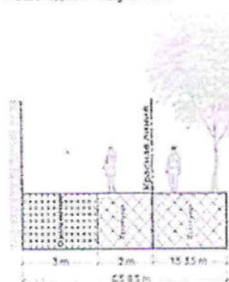
Пешеходный модуль тип 1
