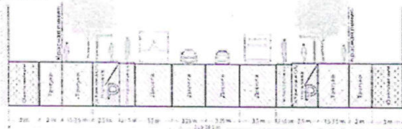
Магистральная улица районного значения тип 2
