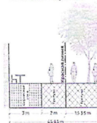
Пешеходный модуль тип 2
