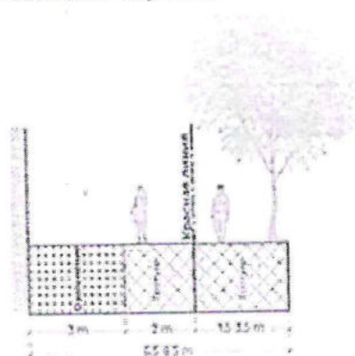
Пешеходный модуль тип 1
